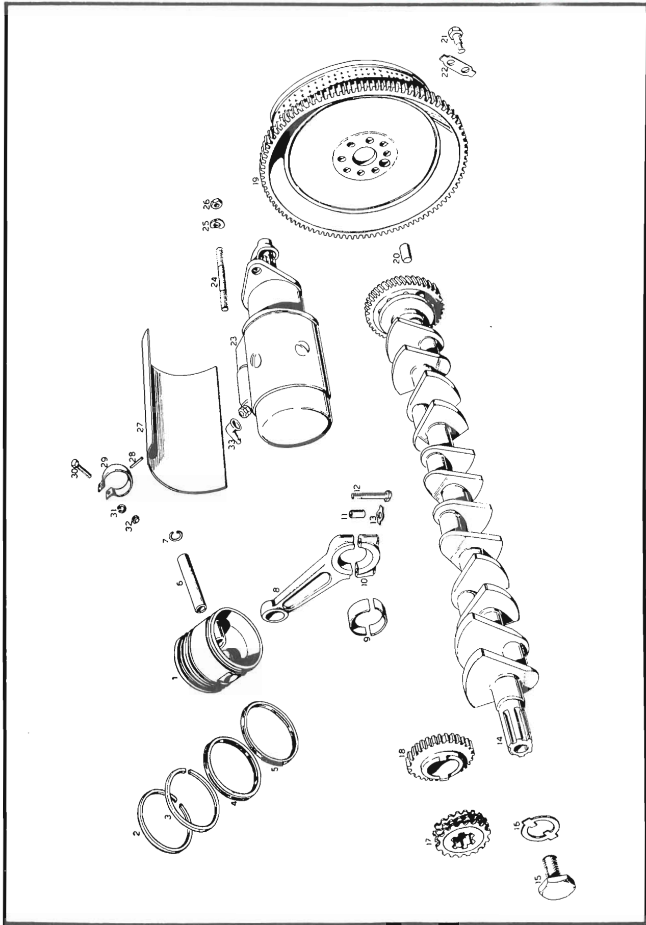
Tavola 3 - Manovellismo, volano e motorino avviamento
